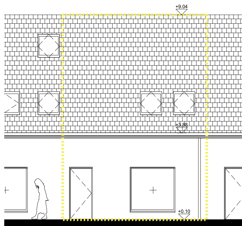
NOORD GEVEL
