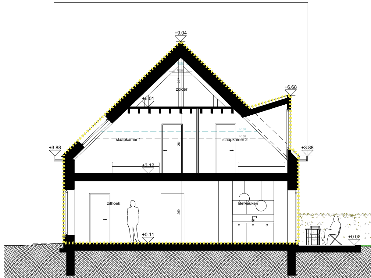
SNEDE A2
